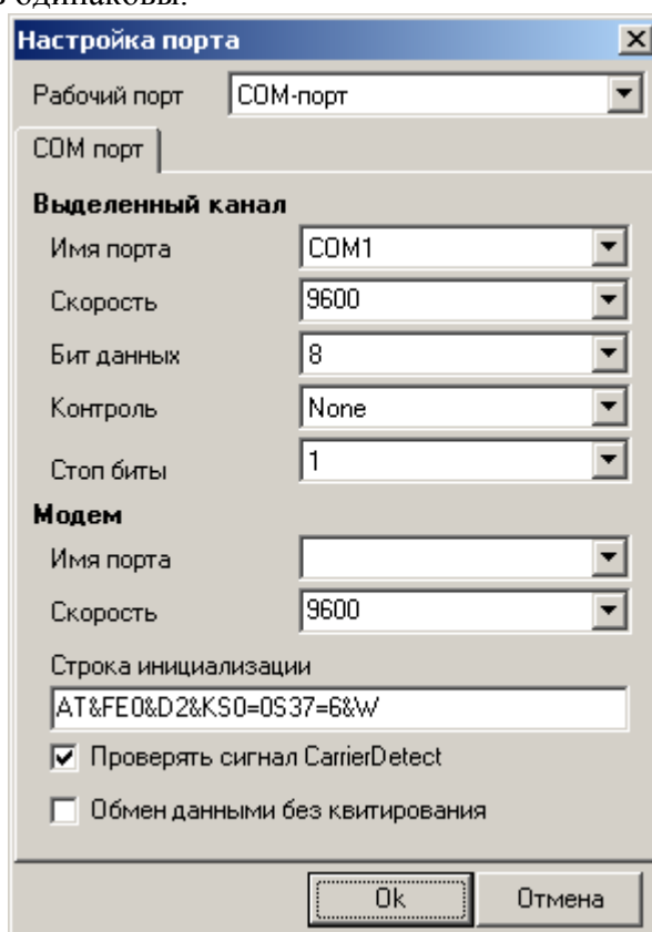
Рисунок 4.19 — Окно настройки COM-порта
